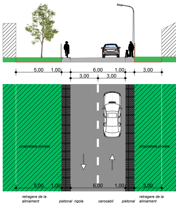
secțiune transversală BB strada Ienuparului
