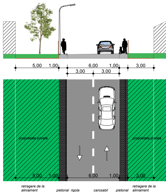
secțiune transversală AA strada Molidului
